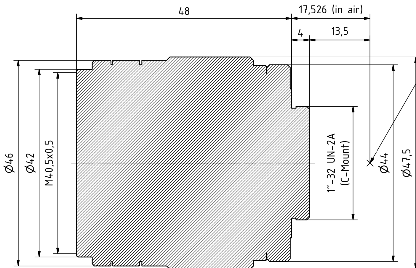
A-A ( 2 : 1 )
