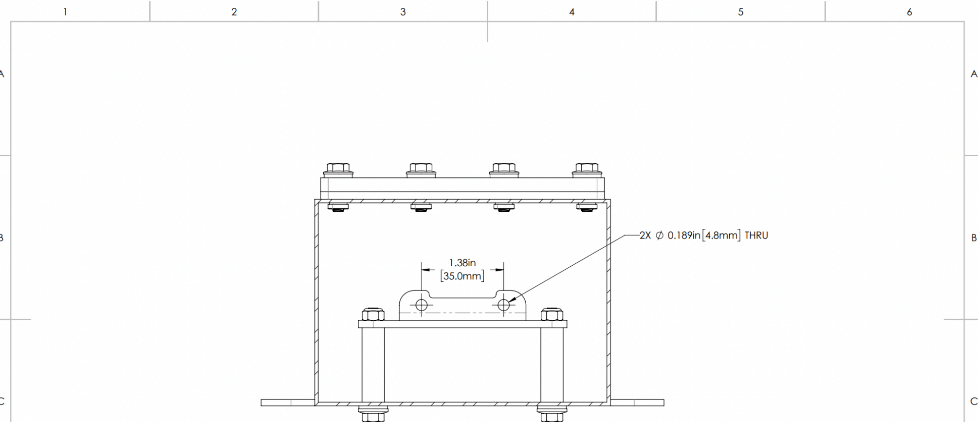
SECTION A-A
