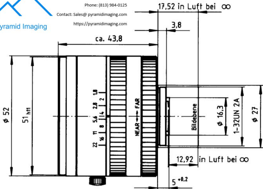
Cinegon 1,8/4,8 in man. Blendenkörper
