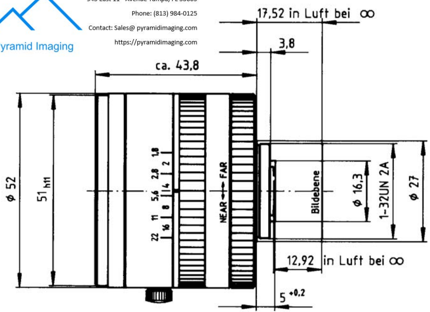
Cinegon 1,8/4,8 in man. Blendenkörper
